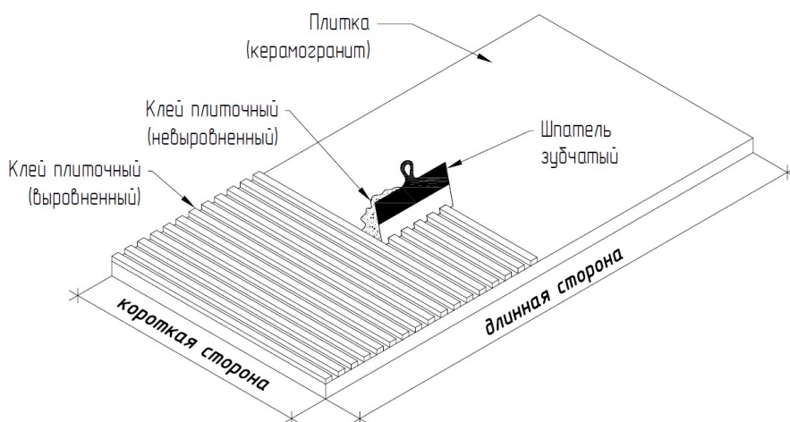
Нанесение плиточного клея на плиту
