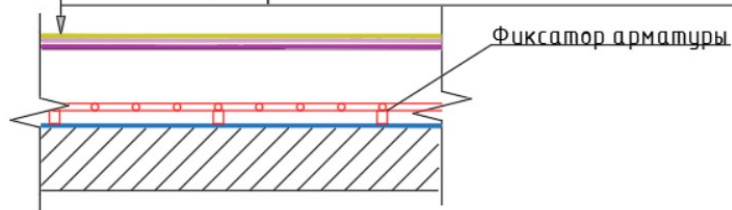
Сечение готового покрытия.
