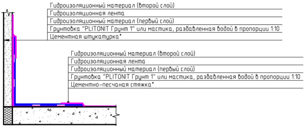
Разрез 1-1
